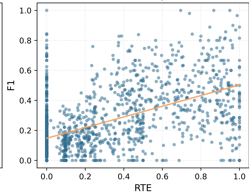
GPTAcc ( \rho=0.3619 , p=0.0000 )
