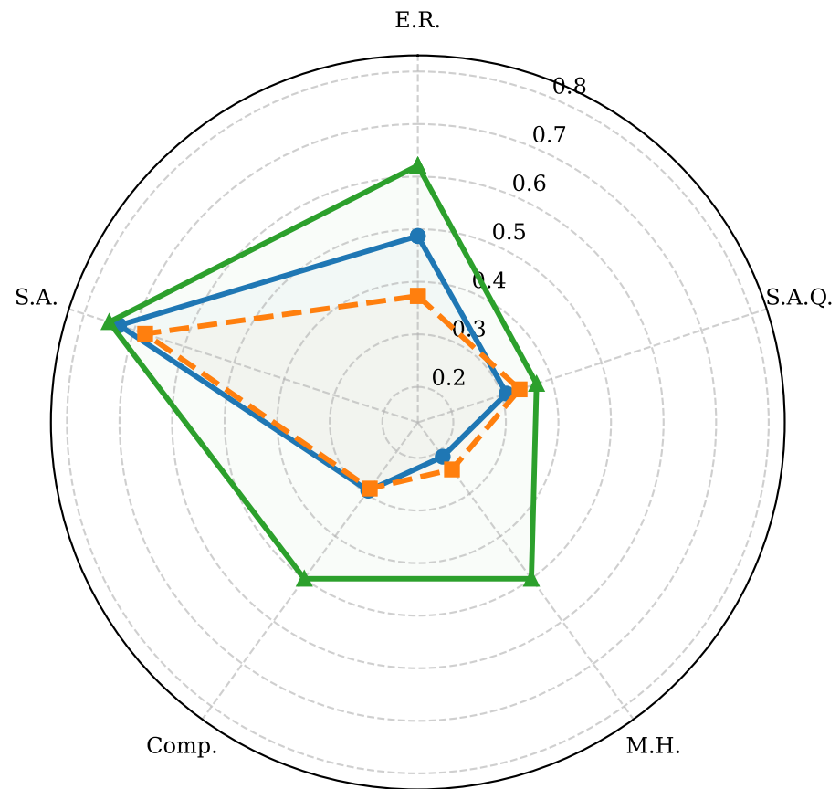
LJ Score
