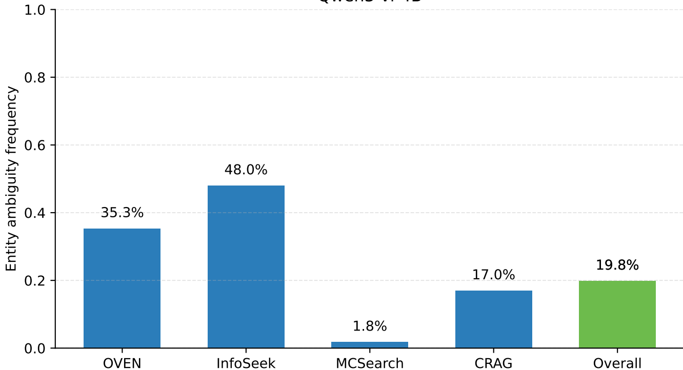
Qwen3-vl-4B
