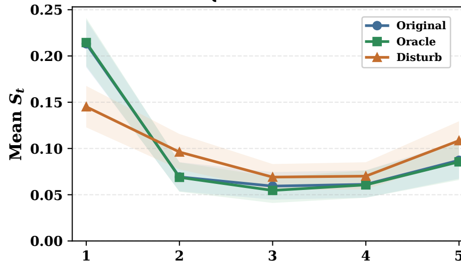
Qwen3-vl-32B
