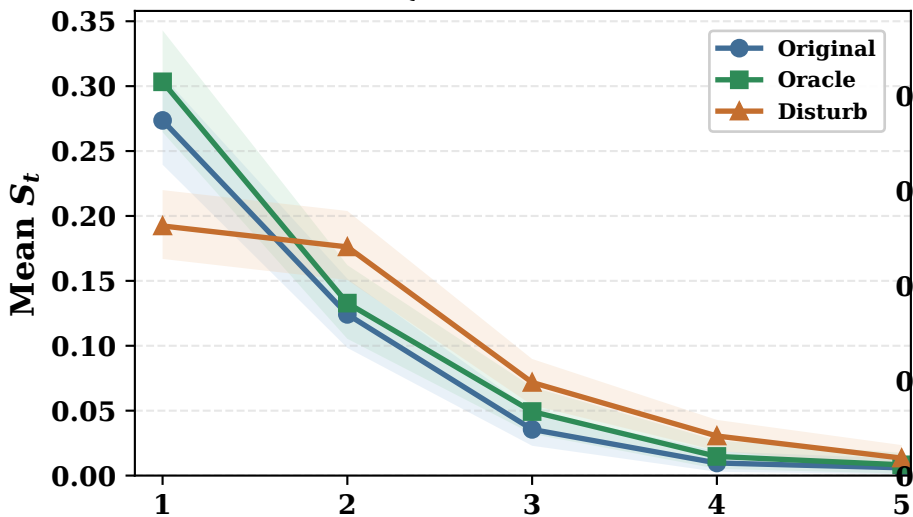
Qwen3-vl-32B
