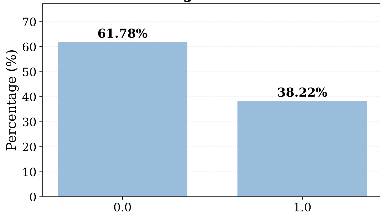
LJ Score
