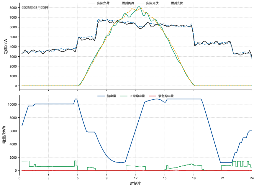
图 6: 2025 年 3 月 20 日 24 小时预测值与实际值
