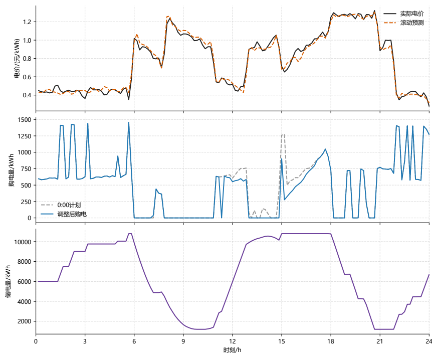
图 16: 2025 年 3 月 20 日价格预测与滚动调度结果
