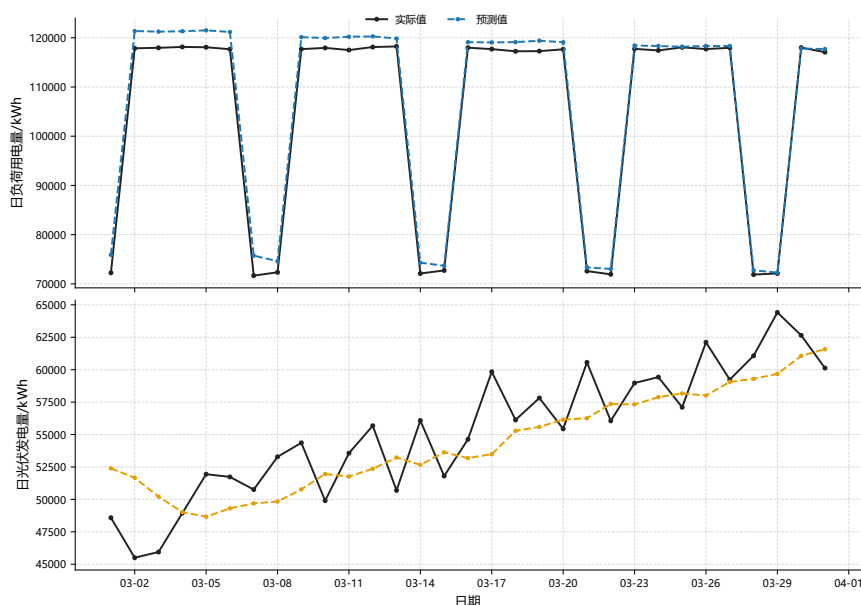
图 7: 2025 年 3 月日总电量的预测值与实际值
