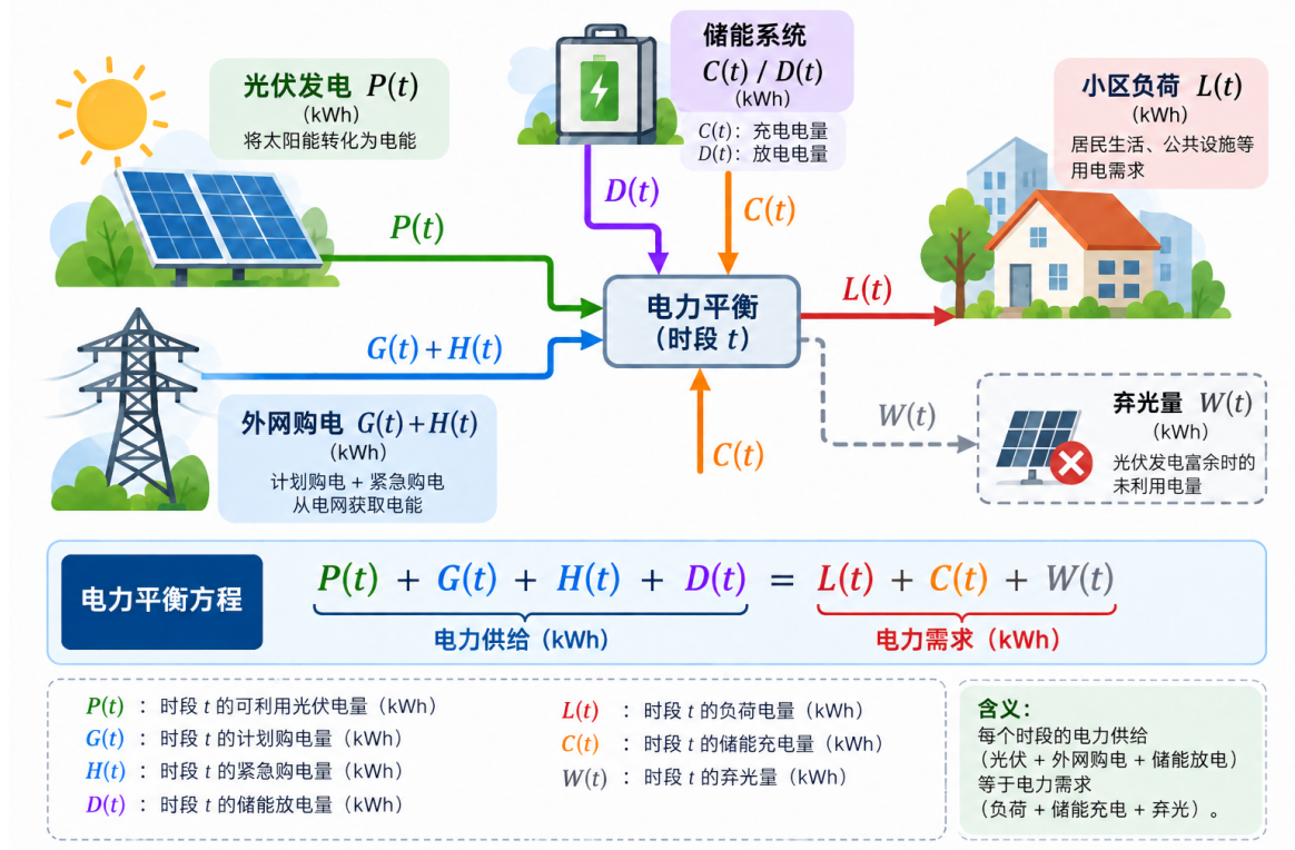
图 1: 贯穿全文的微网电力平衡关系
