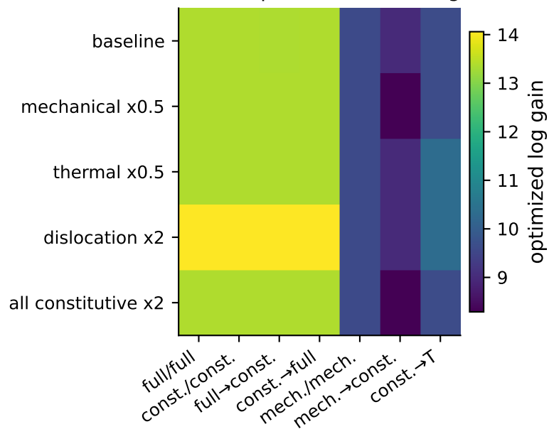
(d) Same-selector frozen-window convergence
