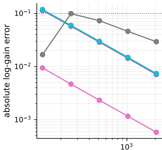
(d) Same-selector frozen-window convergence
