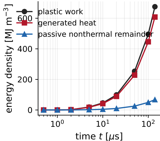
(d) Work-heat-storage partition
