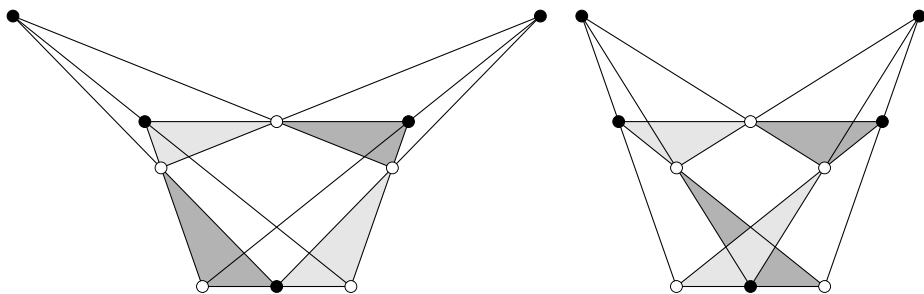
Рис. 14.2. Конфигурация Дезарга — пятиугольники
