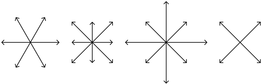
Рис. 14.1. Системы корней A_2 , B_2 , C_2 и D_2 , соответствующие классическим алгебрам Ли \mathfrak{sl}(3) , \mathfrak{o}(5) , \mathfrak{sp}(4) и \mathfrak{o}(4) соответственно
