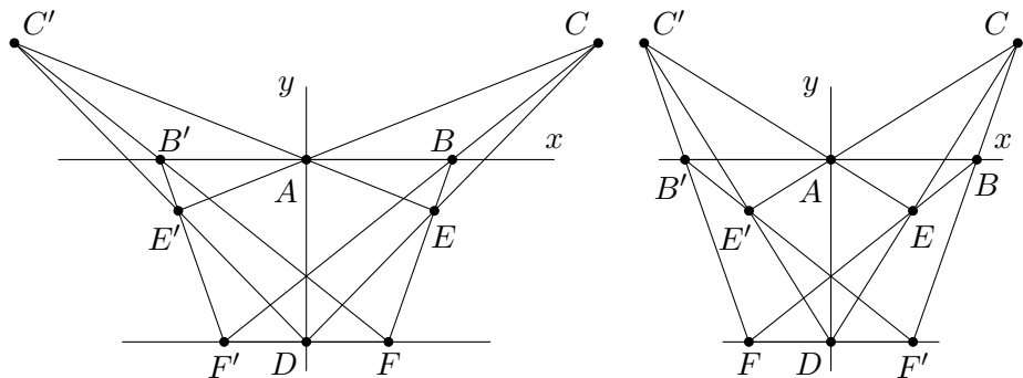
Рис. 14.3. Конфигурация Дезарга — чертежи
