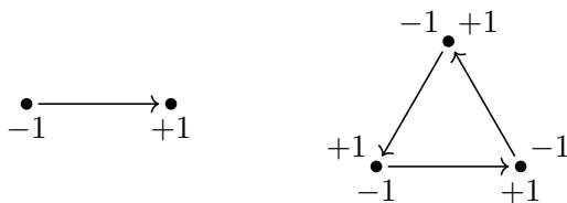
Рис. 14.4. Ориентированные симплексы
