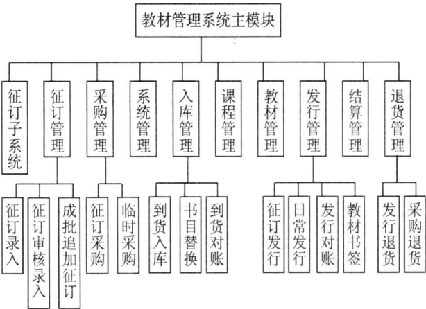
图 2 系统模块结构图
