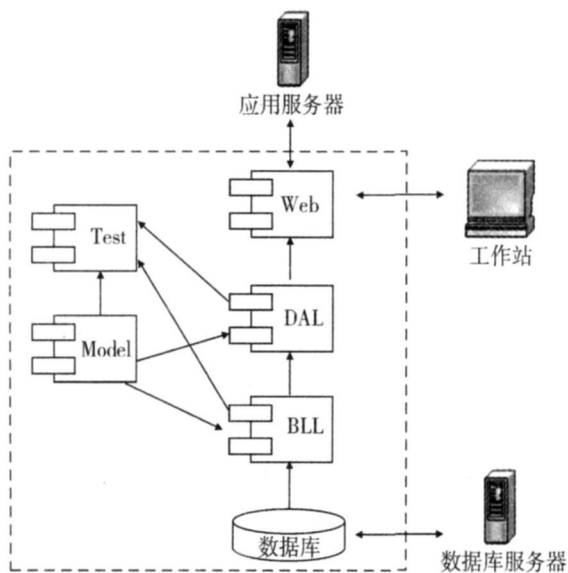
图 1 系统架构图
