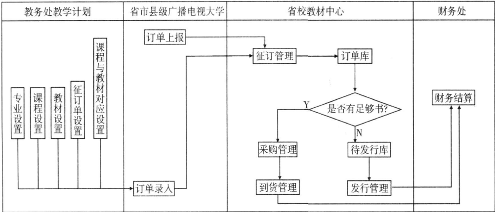
图 3 教材管理系统的流程图
