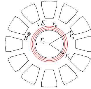
Fig. 9. Brillouin flow in the magnetron.
