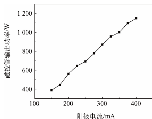
图 5 阳极电流对磁控管输出功率的影响
