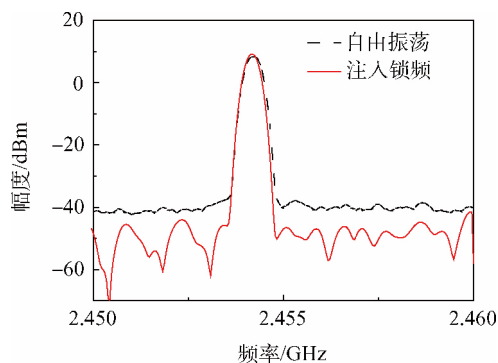
图 6 注入锁频对磁控管输出频谱的影响
