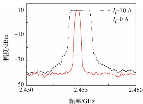
图 4 自由振荡状态下磁控管输出频谱
