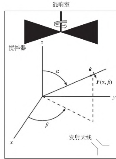
图1 混响室内电场角谱矢量示意图
