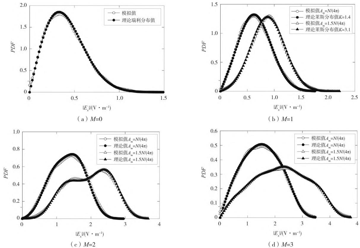
图 2 蒙特卡洛模拟结果
