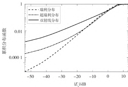
图 3 超瑞利分布的模拟
