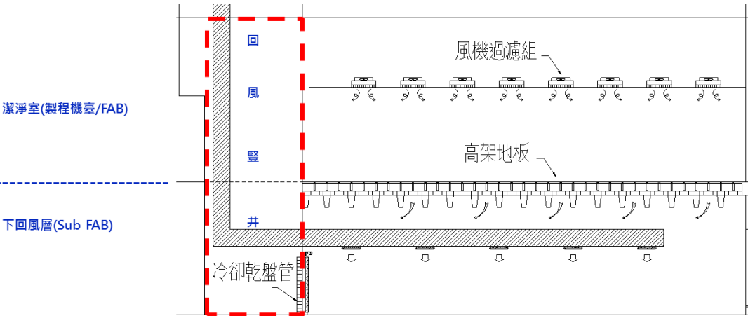
雙層型式潔淨區剖面示意圖之二
