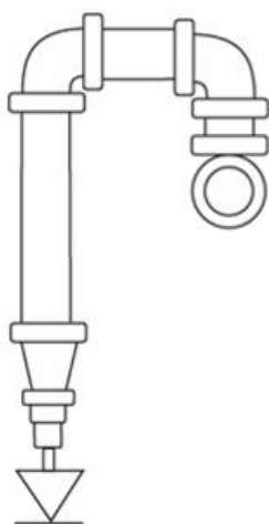
附圖五 撒水頭配管設置回彎管圖例
