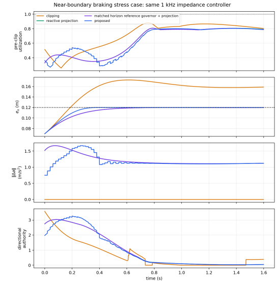
Fig. 3. 近边界制动压力案例。
