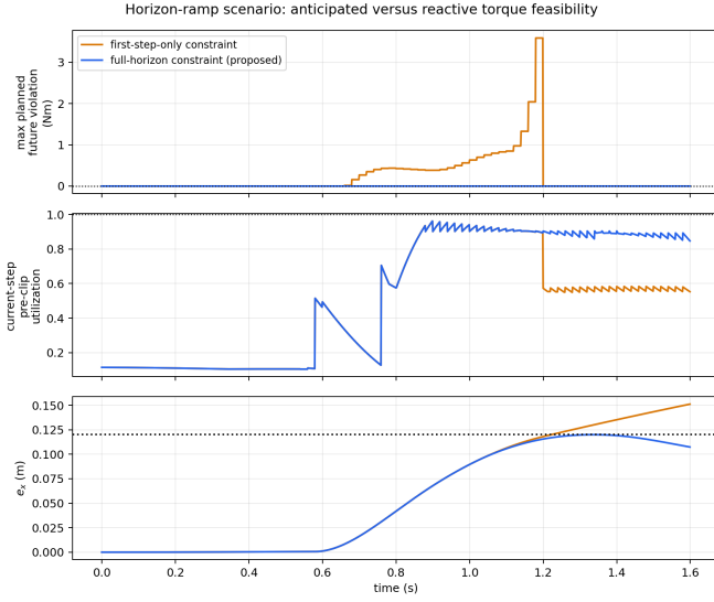
Fig. 1. 时域斜坡场景：仅约束第一步的方案眼见当下合法，却径直走向一个非法的未来；全时域约束方案则提前预见到了这一点。
