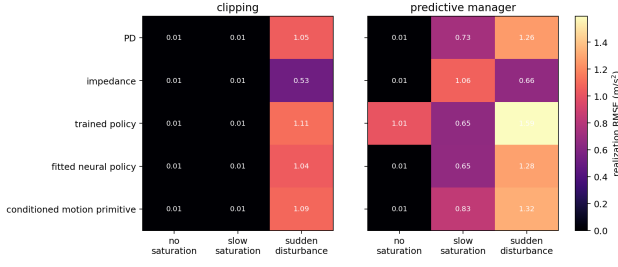
Fig. 4. 五种名义控制器接口下的行为实现残差。
