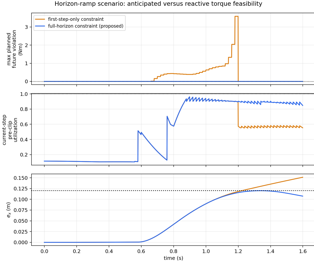
Figure 1: 图 1. 时域斜坡场景：仅约束第一步的方案眼见当下合法，却径直走向一个非法的未来；全时域约束方案则提前预见到了这一点。
