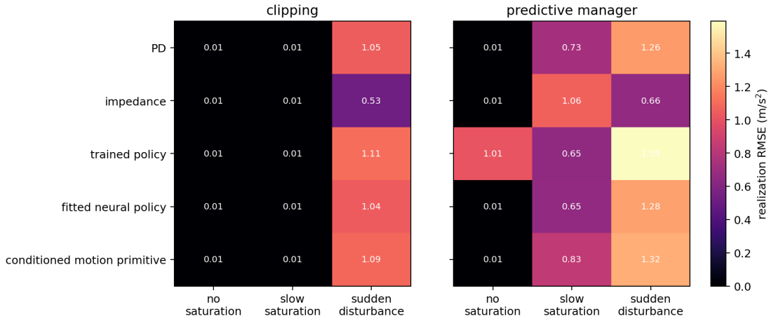
Figure 4: 图 4. 五种名义控制器接口下的行为实现残差。
