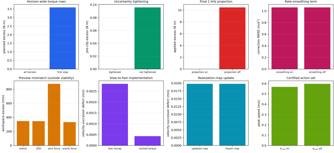
Figure 5: 图 5. 对预测式与快速通道实现选择所做的成对消融实验。
