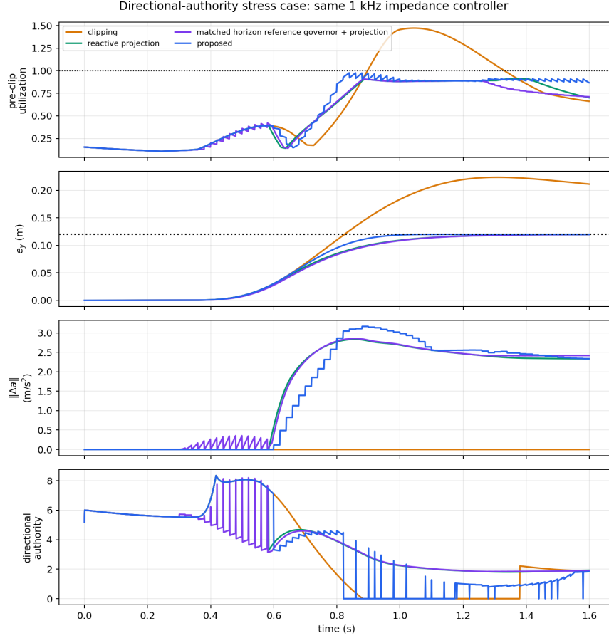
Figure 2: 图 2. 在一个常见阻抗控制器接口下的方向性权限压力案例。
