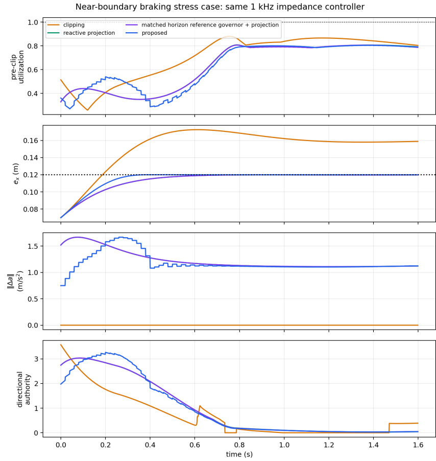
Figure 3: 图 3. 近边界制动压力案例；本文并未从该轨迹推断出任何可行核。
