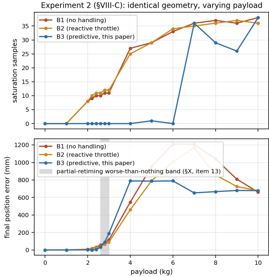
Figure 3: 实验 2 的完整负载扫描：饱和样本数（上）与最终位置误差（下）随负载的变化，三个基线均已给出。阴影带标出 2.6–3.0kg 区间，在此区间内 B3 的部分重新定时反而使最终误差比 B1 未经修改的基线更差——即上文的第一项发现。
