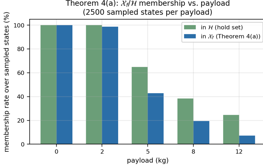
Figure 1: \mathcal{H} 与 \mathcal{X}_f 的成员率随负载的变化，每个负载级别下对 2500 个均匀采样的构型（对 \mathcal{X}_f 还包括可制动盒内的速度）求得。
