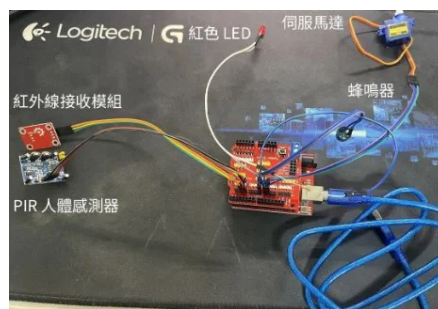
▲ 紅外線、PIR、蜂鳴器與伺服馬達
