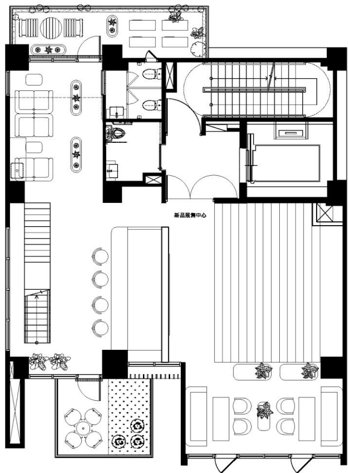
七層平面圖 H=420cm
