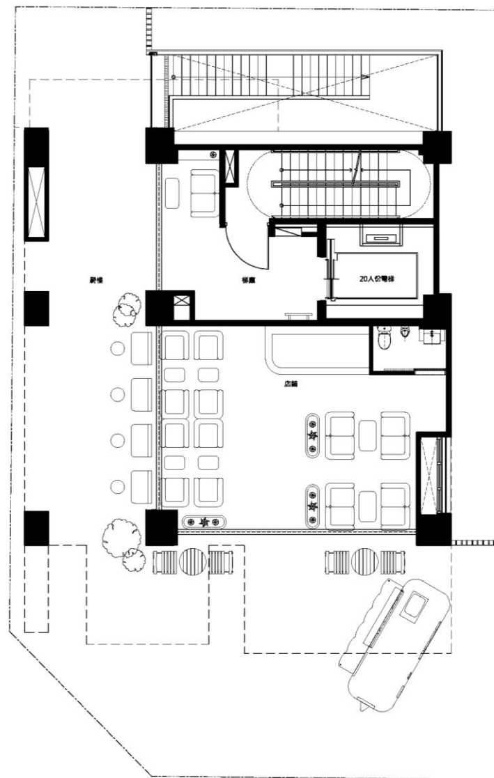
一層平面圖 H=425cm
