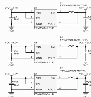
电源
