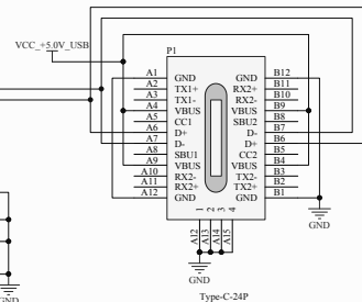
Type-C接口
