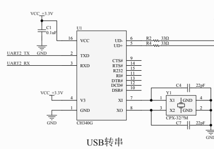
USB转串
