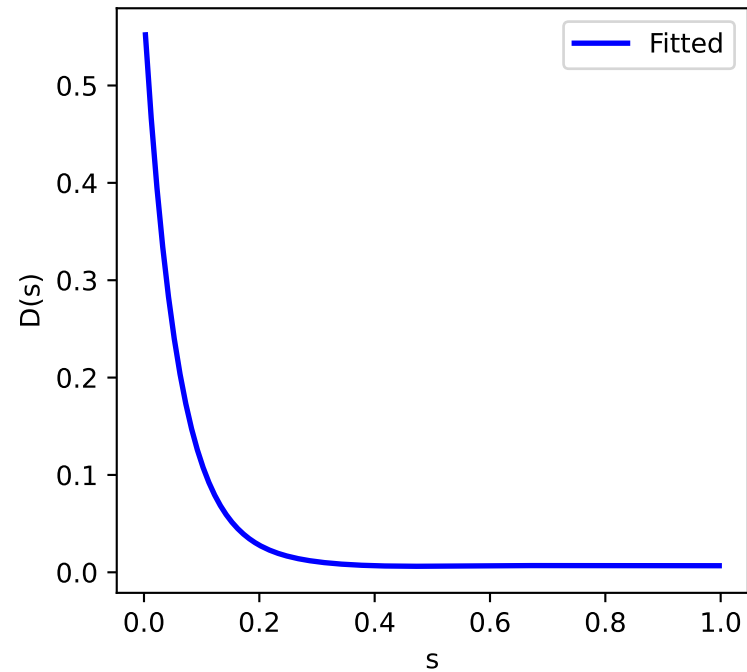
Diffusion
