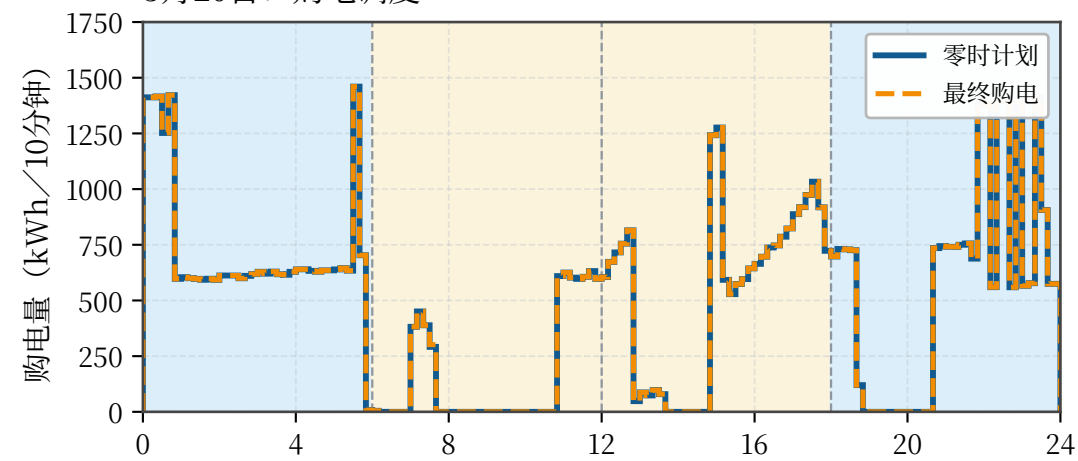
3月20日：购电调度
