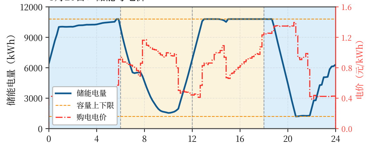
3月20日：储能与电价
