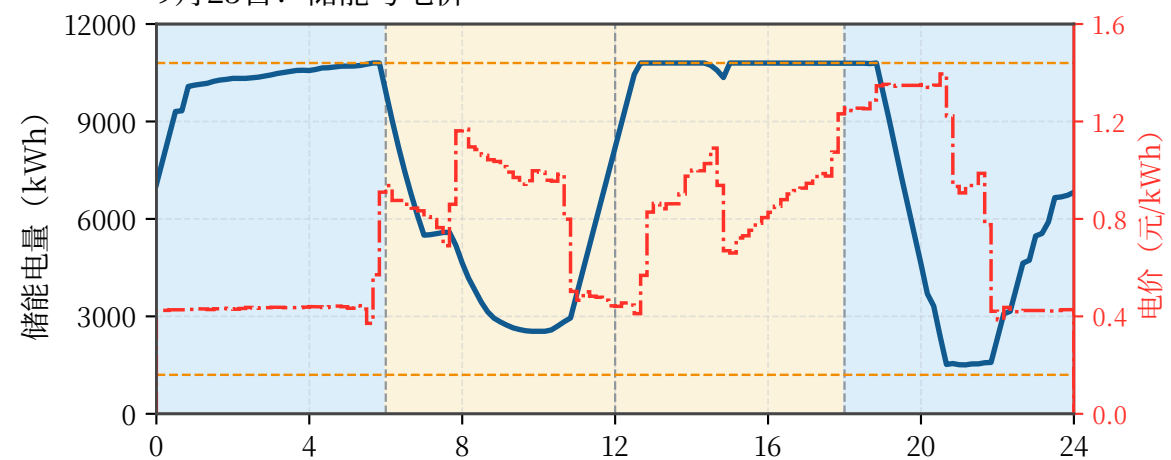
9月23日：储能与电价
