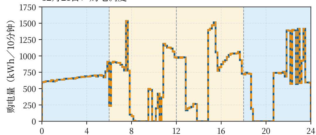
12月21日：购电调度
