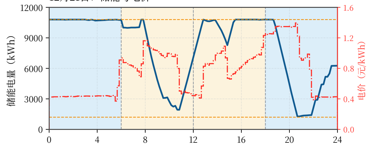
12月21日：储能与电价
