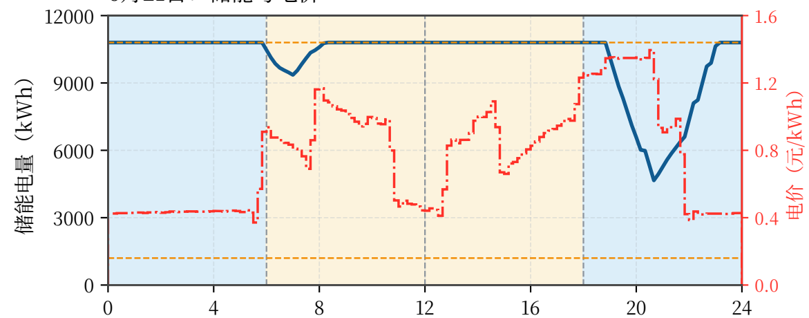
6月21日：储能与电价
