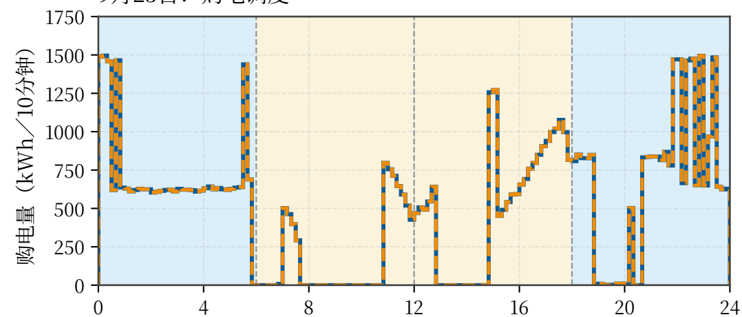
9月23日：购电调度
