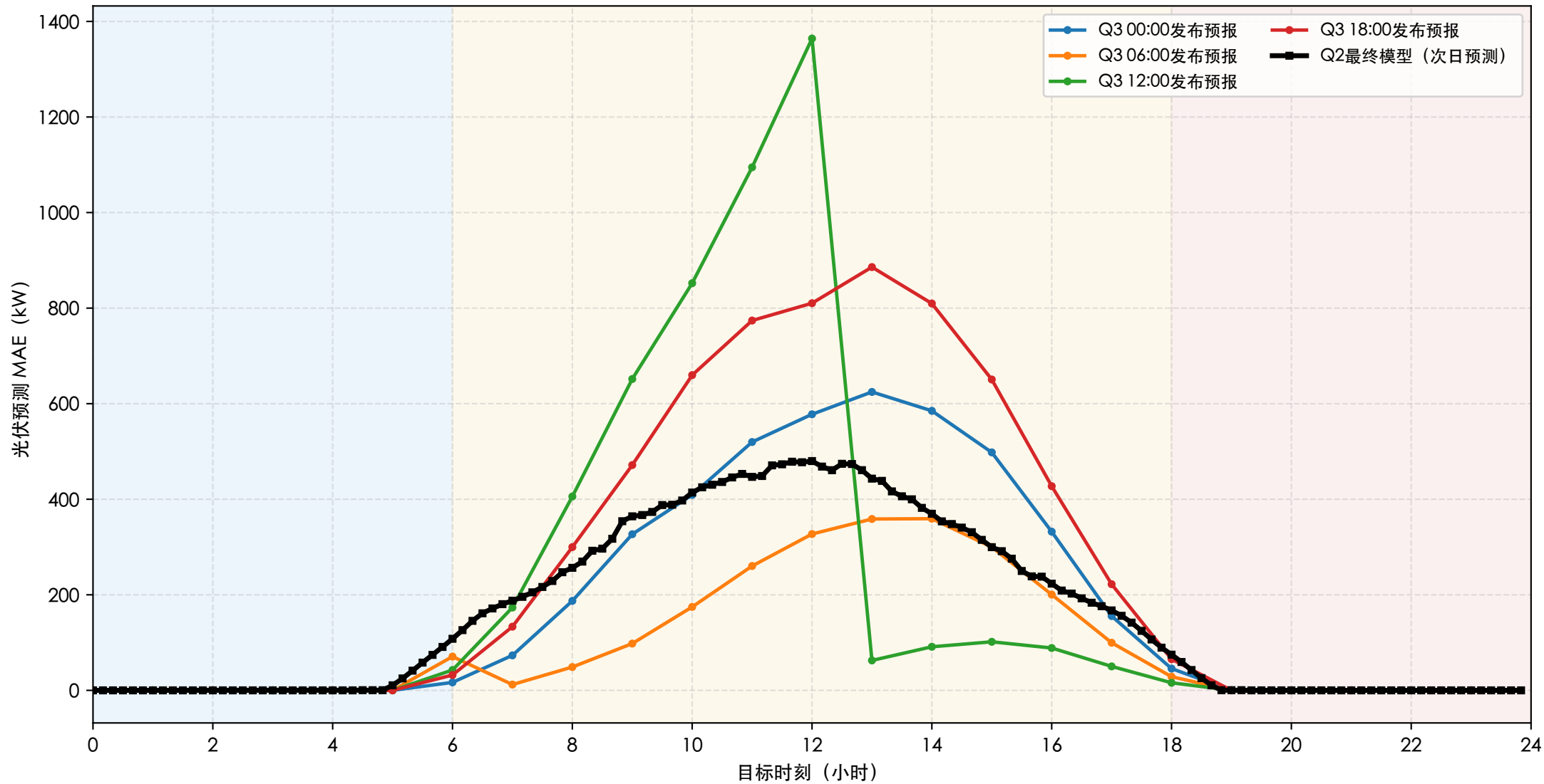
Q2最终模型与Q3各版本光伏预测误差的目标时刻对比
