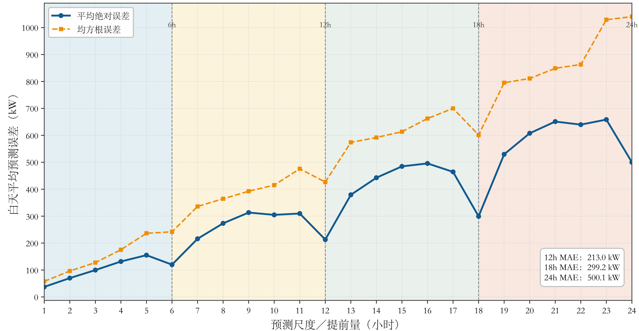
光伏预测误差随预测尺度的变化（白天 06:00--18:00）
