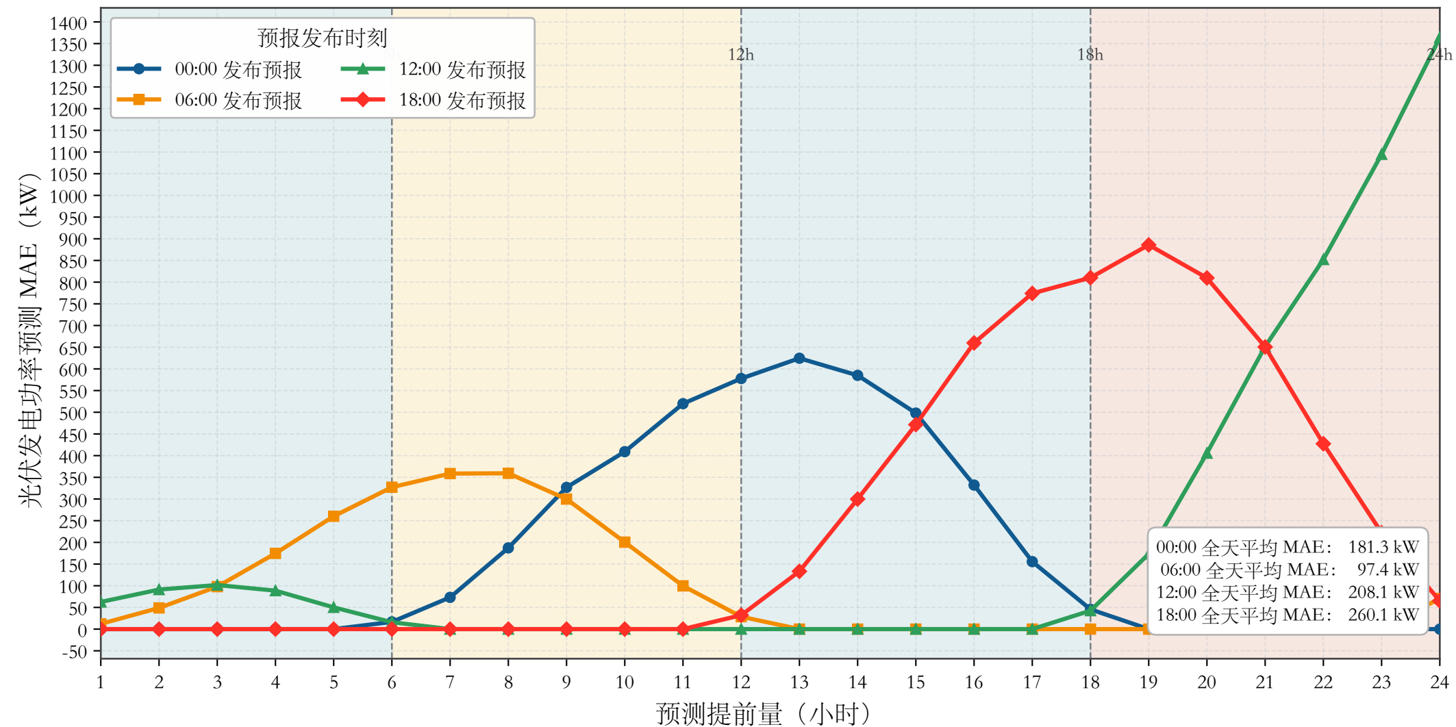
不同发布时刻的光伏预报误差随预测提前量的变化 (2025 全年全天)
