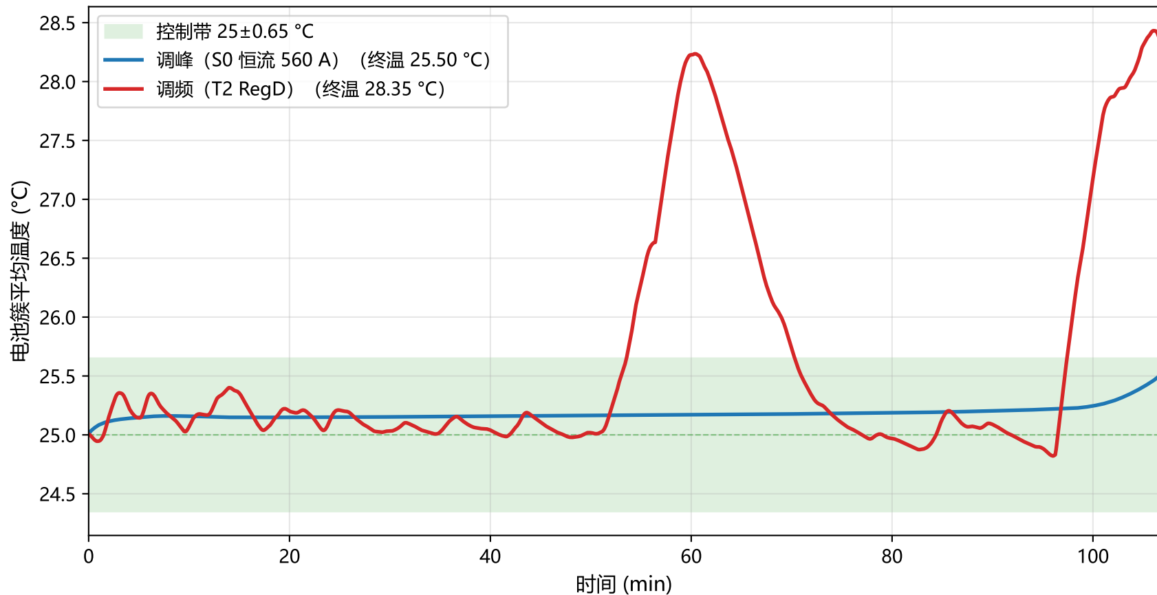
调峰与调频工况：NMPC 电池簇平均温度曲线
