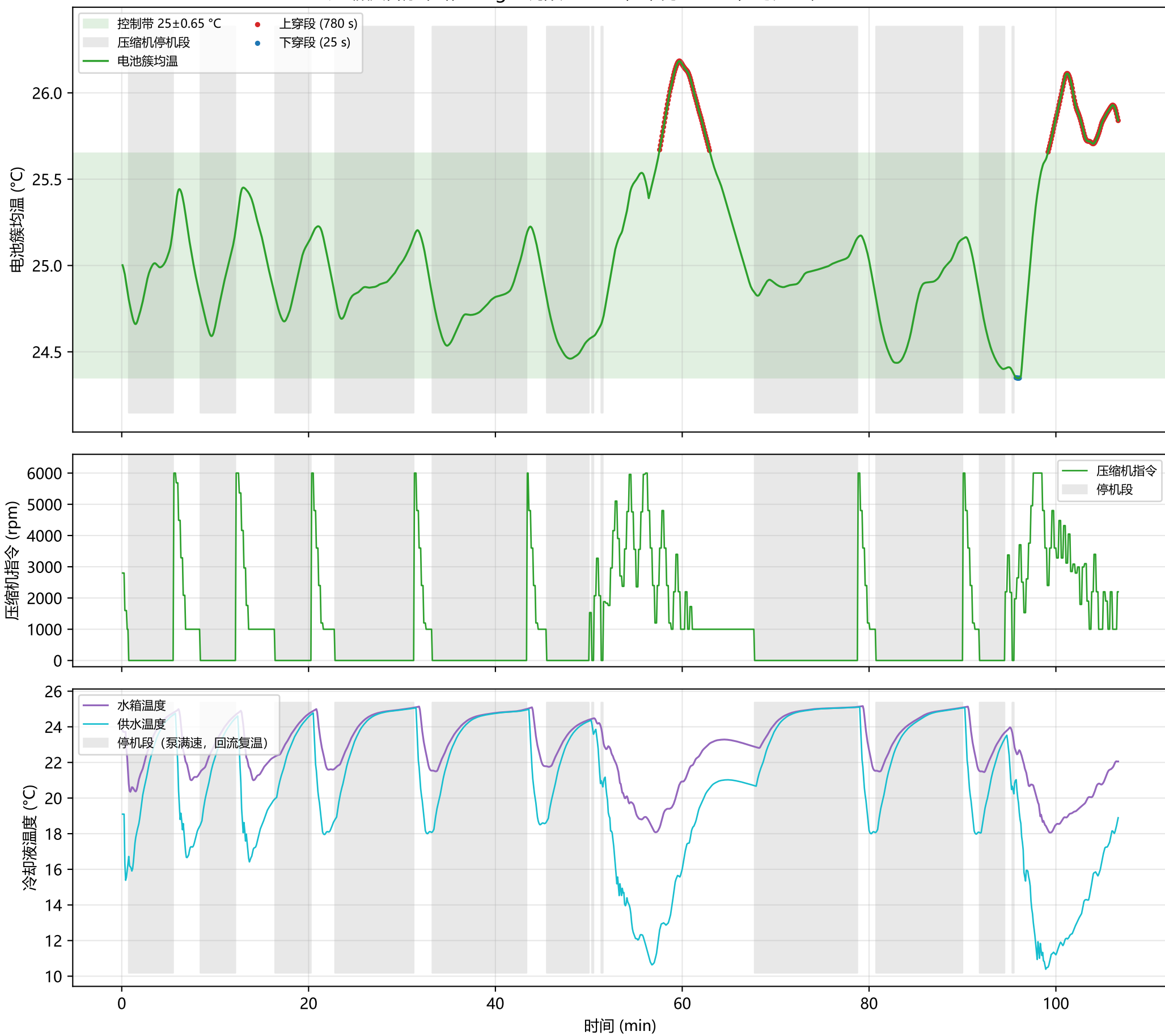
8D4d 压缩机启停策略：RegD 调频 6400 s，带内 87.4%，均温全程 24.35~26.18 °C
