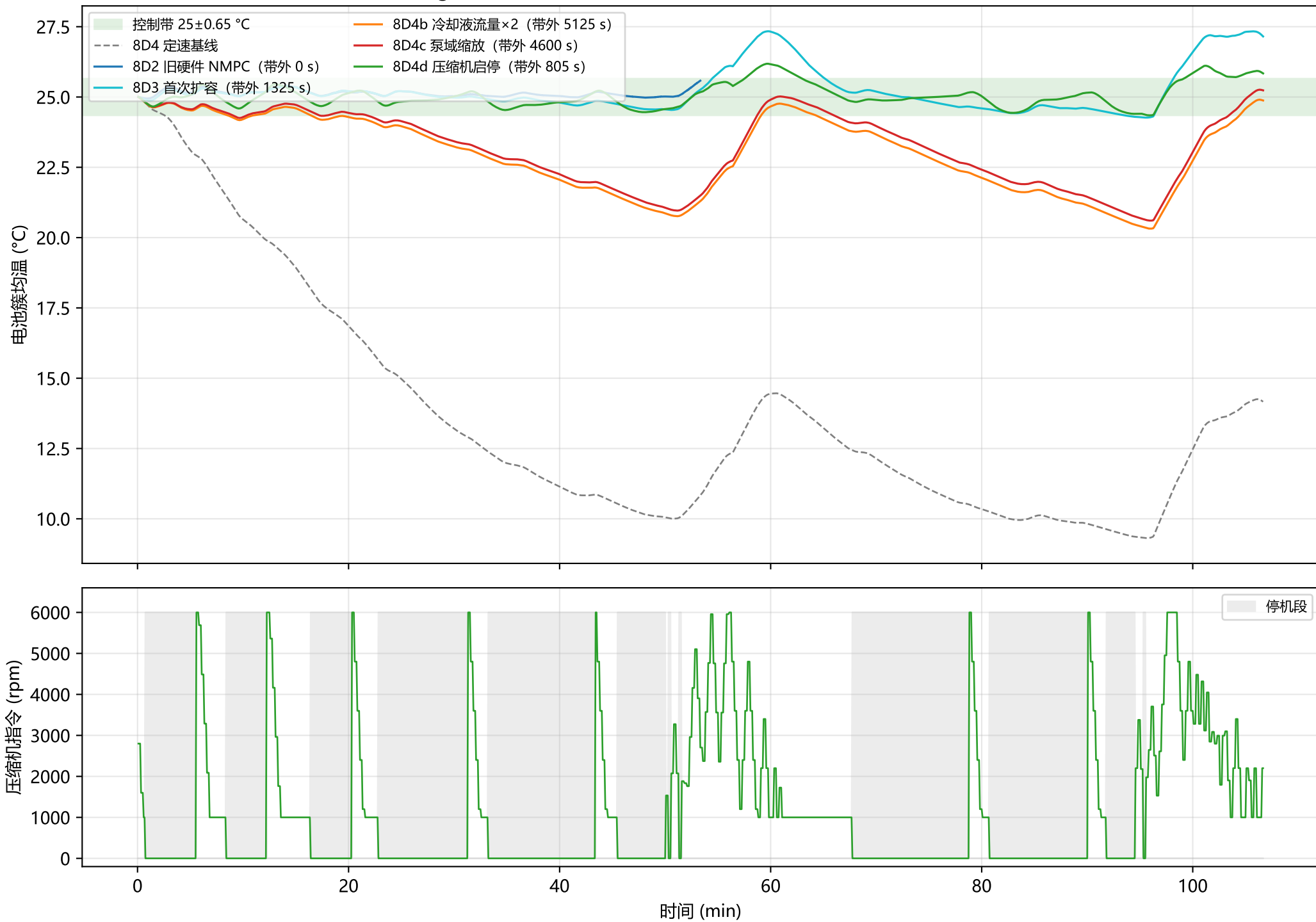
RegD 调频工况：五代硬件/控制演进的温度对比 (T2, 6400 s)
