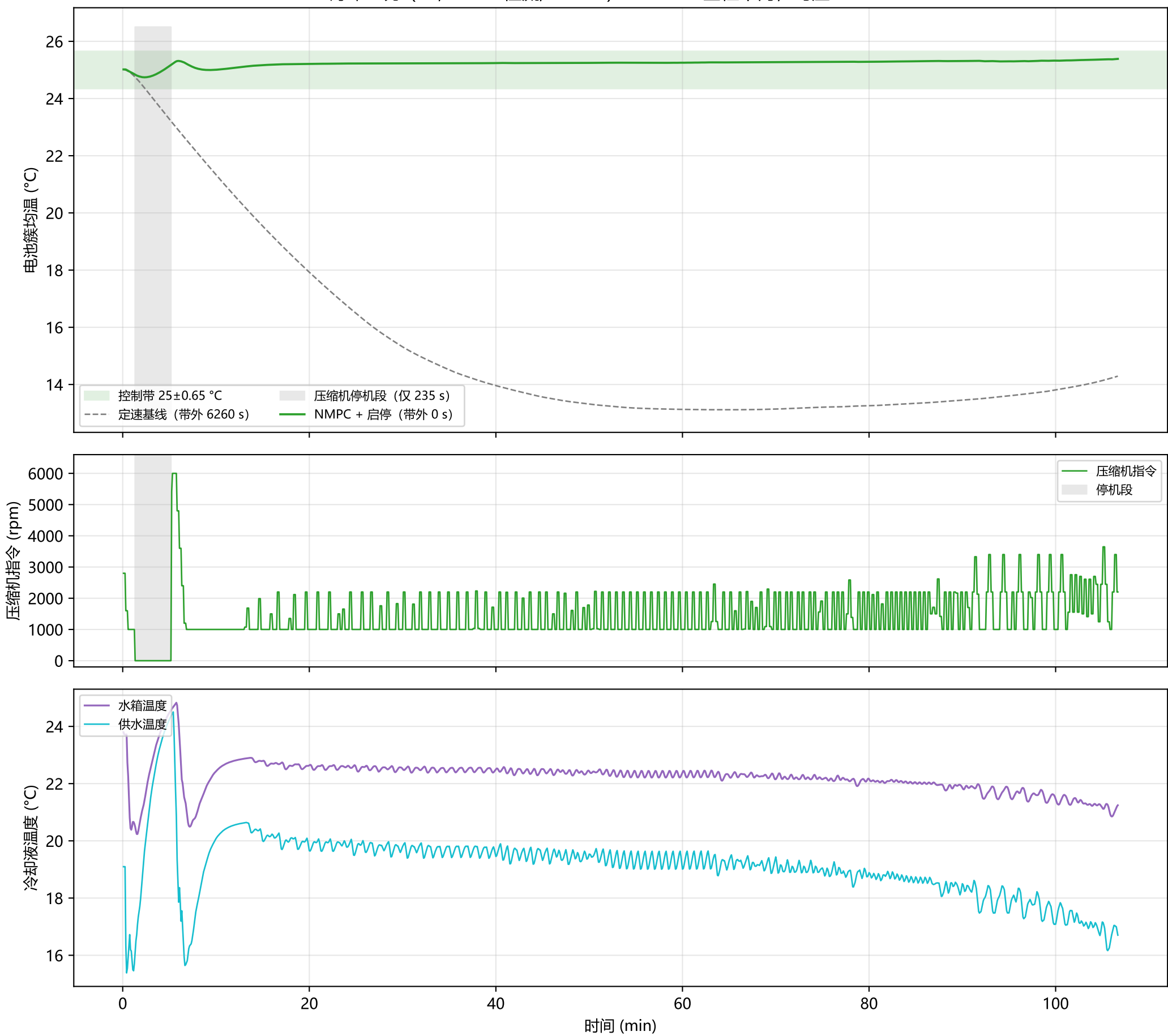
8D4d 调峰工况 (S0, 560 A 恒流, 6400 s) : NMPC 全程带内, 均温 24.74~25.39 °C
