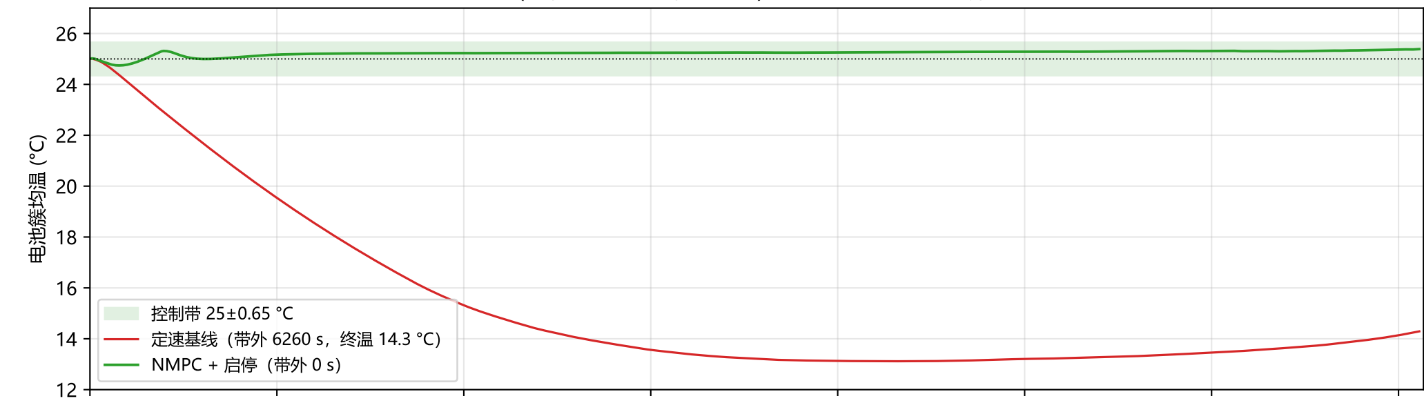
8D4d 调峰工况 (S0, 560 A 恒流, 6400 s) : 定速基线严重过冷, NMPC 全程带内
