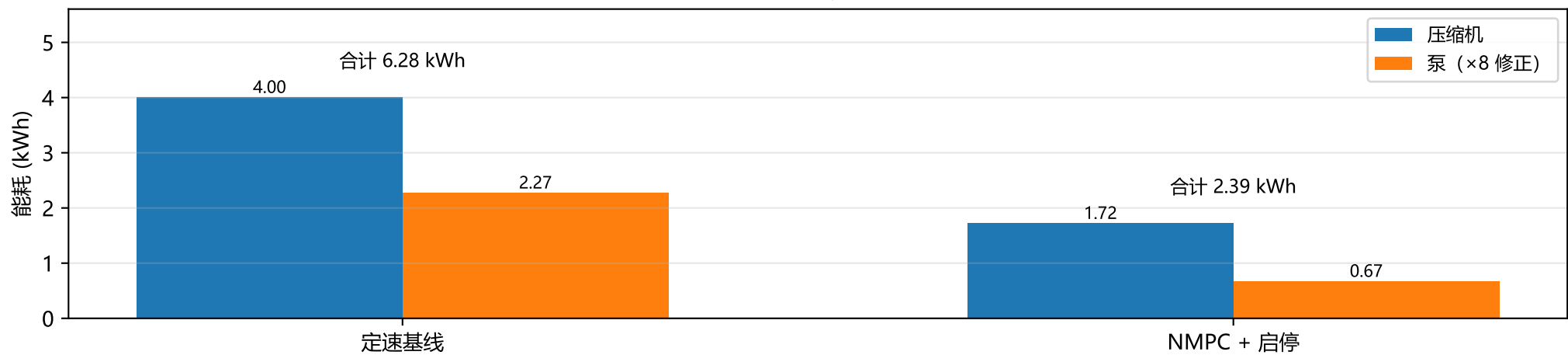
NMPC 总能耗 2.39 kWh, 较定速基线节省 62%
