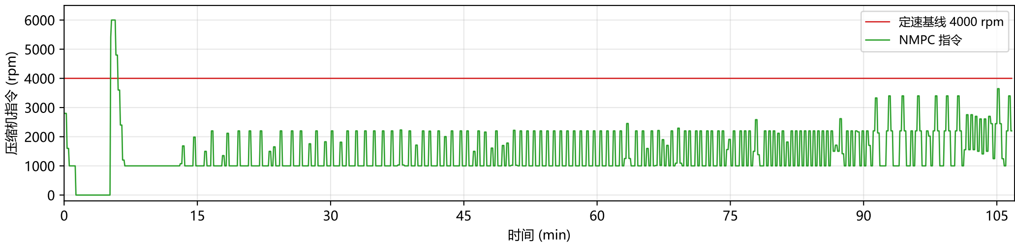
NMPC 总能耗 2.39 kWh, 较定速基线节省 62%
