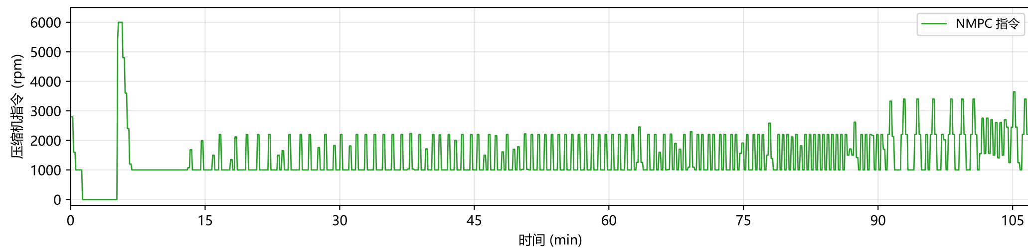
NMPC 总能耗 2.39 kWh, 较定速基线节省 62%
