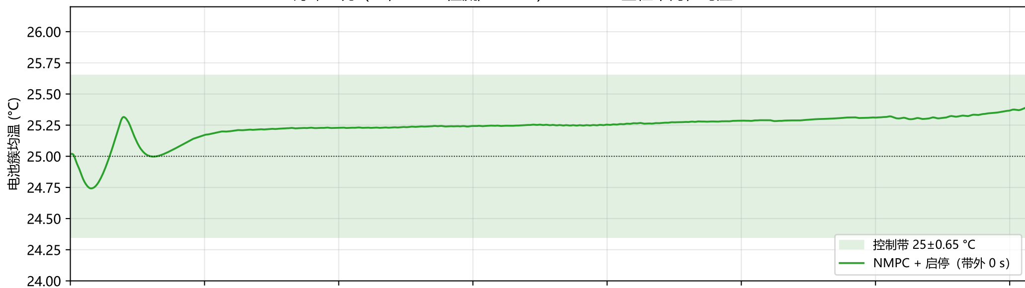
8D4d 调峰工况 (S0, 560 A 恒流, 6400 s) : NMPC 全程带内, 均温 24.74~25.39 °C
