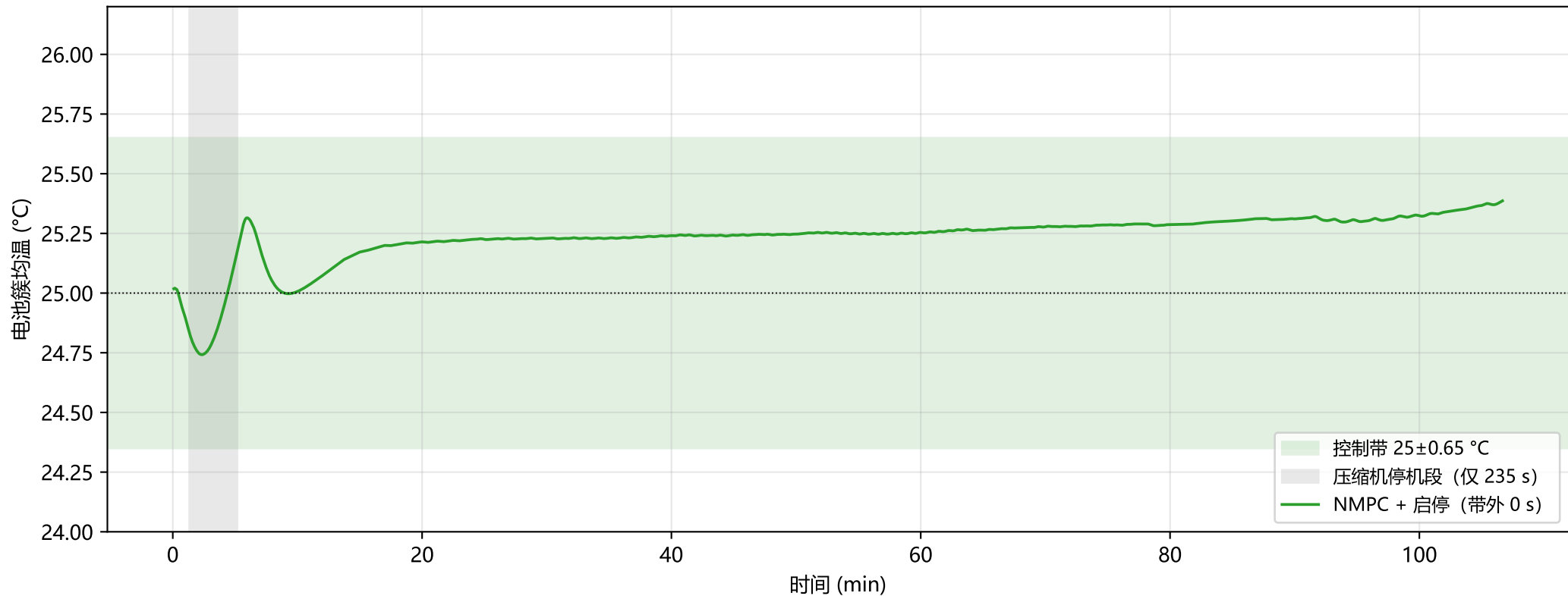
8D4d 调峰工况 (S0, 560 A 恒流, 6400 s) : NMPC 全程带内, 均温 24.74~25.39 °C
