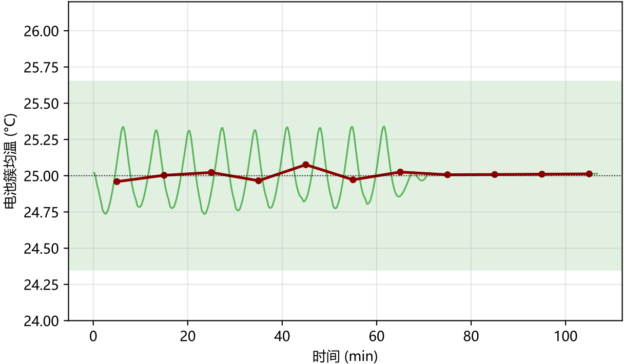
8D4f (簇口径修正 + 重锚定) : 末 1000 s 均温 25.01 °C (偏差 +0.01 K) , 带外 0 s
