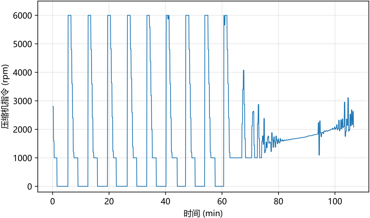
末 1000 s 指令: 均值 2014 rpm, 波动 1095~3106
