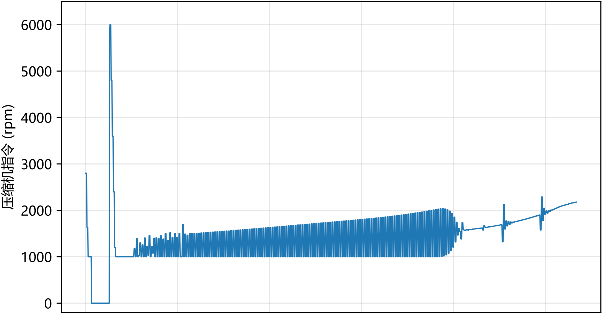
末 1000 s 指令: 均值 1912 rpm, 波动 1322~2289
