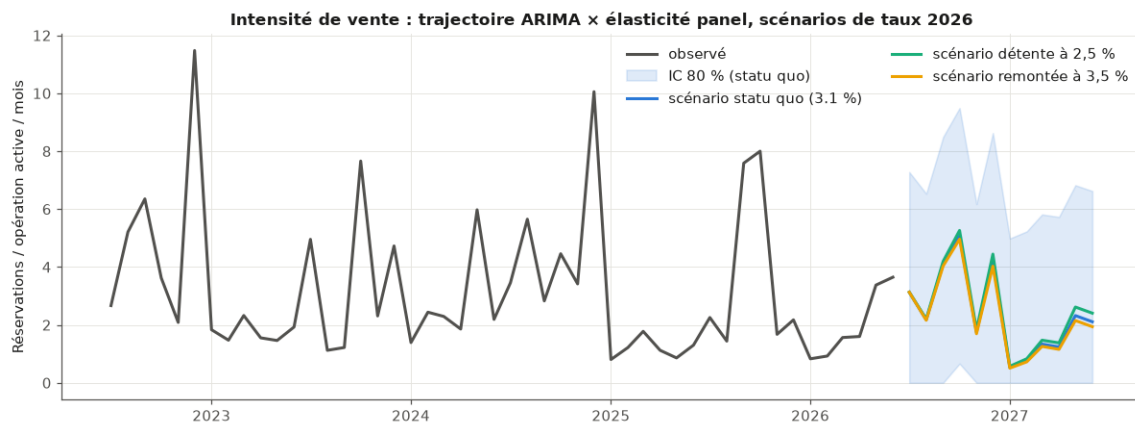
FIGURE 3.4 – Prédiction d'intensité de vente à douze mois sous trois scénarios de taux 2026, avec intervalle à 80 %
