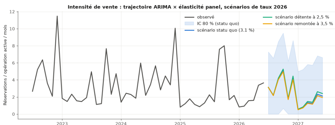
FIGURE 2.4 – Prévvision d’intensité de vente à douze mois sous trois scénarios de taux 2026, avec intervalle à 80 %
