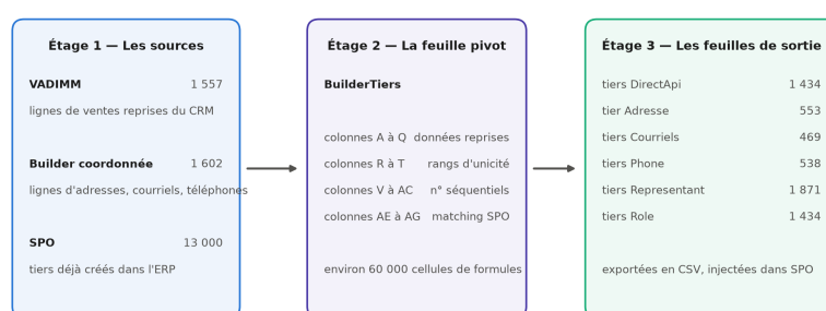
FIGURE 1.3 – La chaîne de traitement à trois étages du fichier de travail
