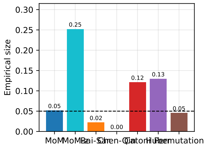
t(10) noise
