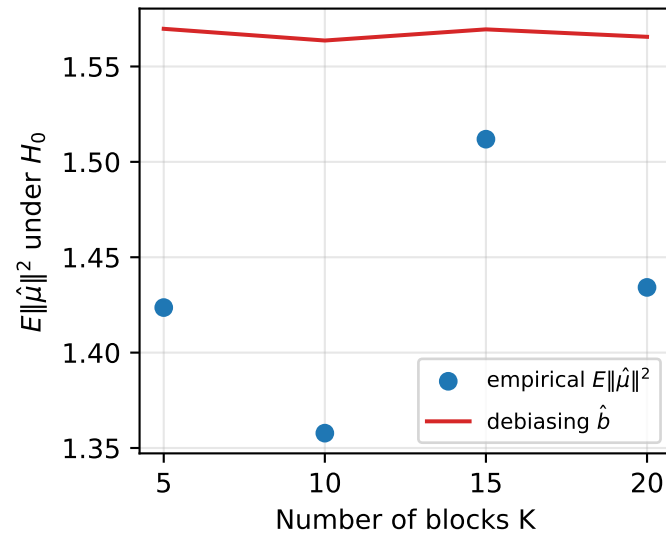
t(10) noise
