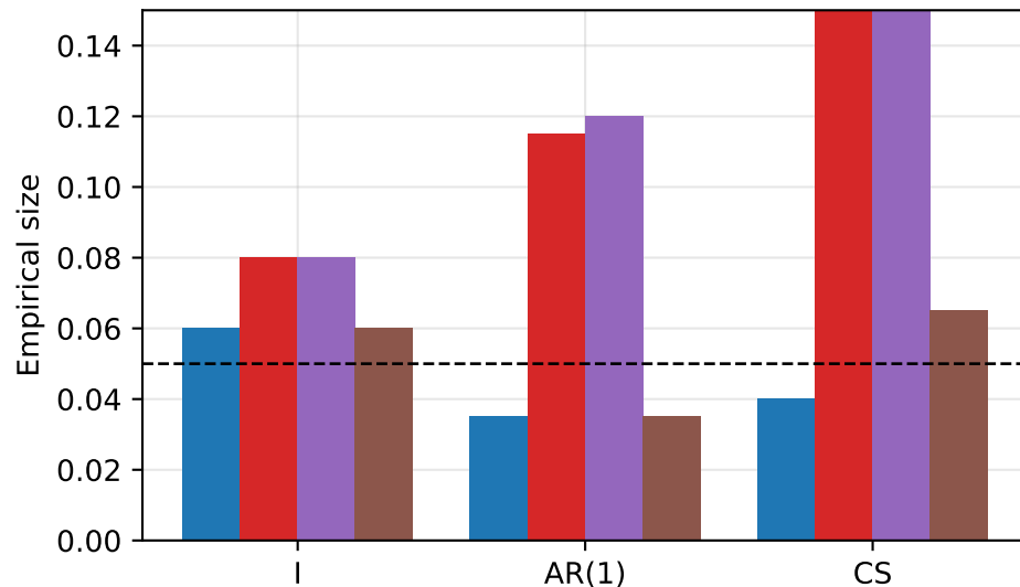
t(10) , p=200 , n=100
