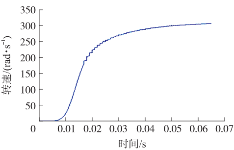
图 7 转速曲线
