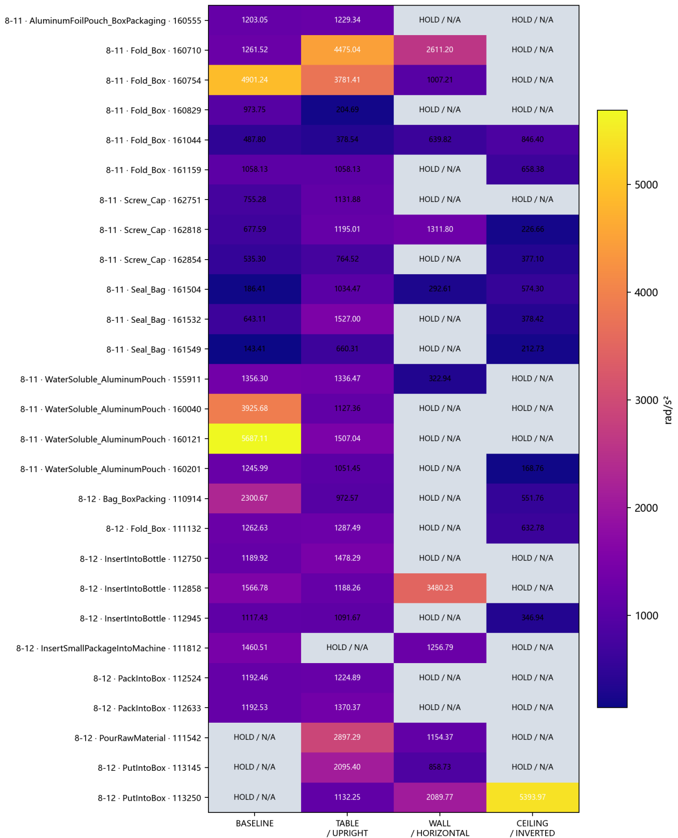
原始节奏最大关节加速度
