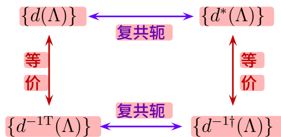
图 9.1: 四个 Lorentz 群 2 维表示之间的关系。
