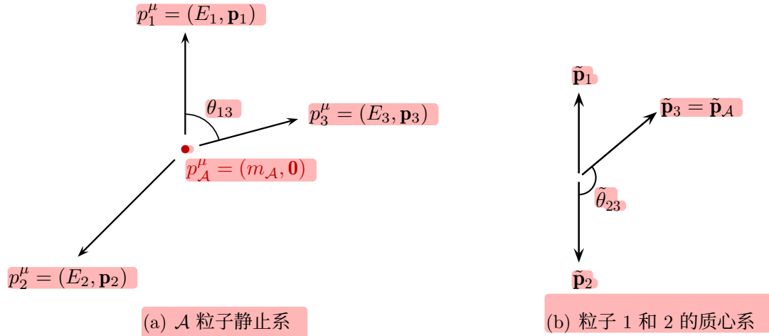
图 6.6: 三体衰变过程的动量示意图, 箭头指示三维动量的方向。
