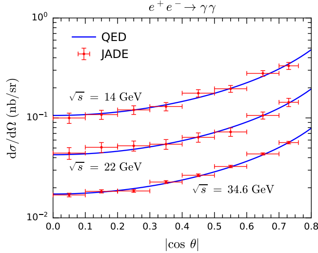
图 8.16: e^+e^- \rightarrow \gamma\gamma 微分散射截面。实验数据来自 JADE 合作组 [43]。
