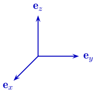
三维矢量空间基底
