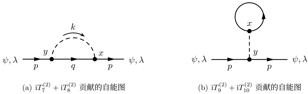
图 7.8: \psi 粒子的单圈自能图。
