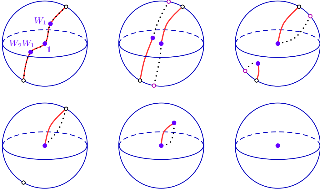
图 3.8: 对闭合曲线连续形变以消除偶数次对径点跳跃并收缩成恒元一点示意图。第一幅图沿同一闭合路径走了两遍, 第一遍用实线表示, 第二遍用点线表示。
