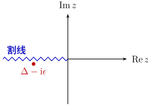
图 12.3: 复平面上 \ln z 的割线和 z = \Delta - i\epsilon 的位置。
