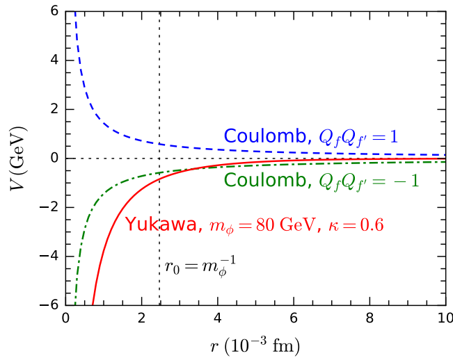
图 8.10: Coulomb 势能与 Yukawa 势能随距离 r 的变化。
