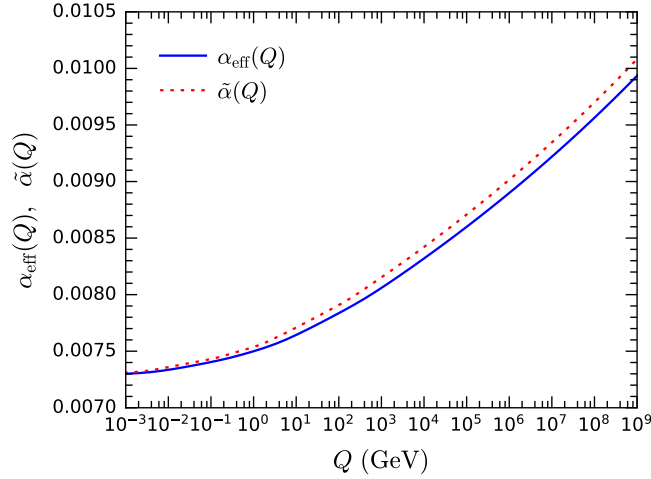
图 12.9: 单圈真空极化图贡献的有效精细结构常数 \alpha_{\text{eff}}(Q) 和重整化精细结构常数 \tilde{\alpha}(Q) 随能标 Q 的跑动。
