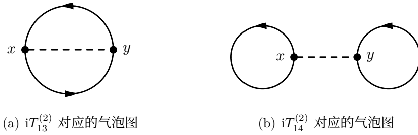
图 7.11: iT_{13}^{(2)} 和 iT_{14}^{(2)} 对应的气泡图。
