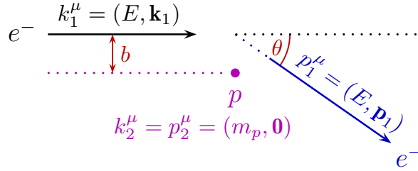
图 8.7: 当入射电子动量远小于 m_p 时, e^- p \rightarrow e^- p 过程的动量示意图, 其中单箭头表示三维动量的方向。
