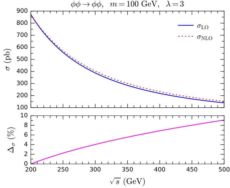
图 12.4: \phi\phi \rightarrow \phi\phi 过程的领头阶 (LO) 和次领头阶 (NLO) 散射截面随质心能 \sqrt{s} 的变化曲线 (上方分图)。下方分图展示了次领头阶与领头阶截面之间的相对偏差。
