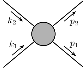
图 8.12: 2 \rightarrow 2 散射过程四维动量示意图。
