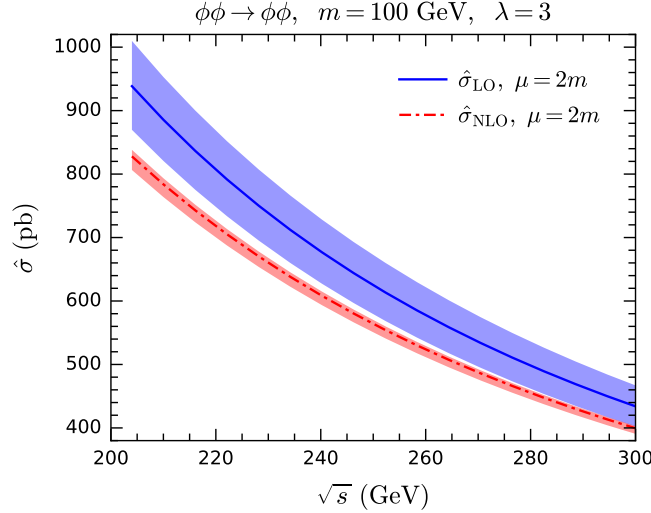
图 12.7: \overline{\text{MS}} 方案中领头阶和次领头阶散射截面对重整化能标 \mu 的依赖性。
