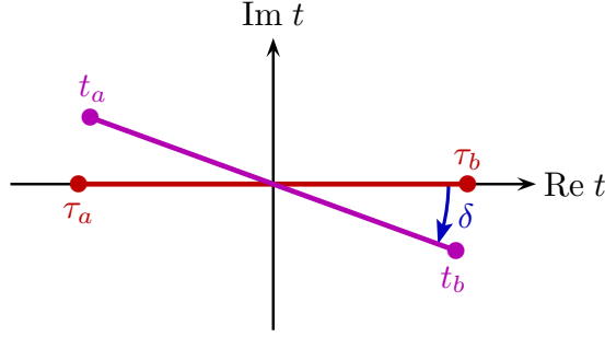
图 11.2: 在 t 的复平面上顺时针转动 \delta 角。
