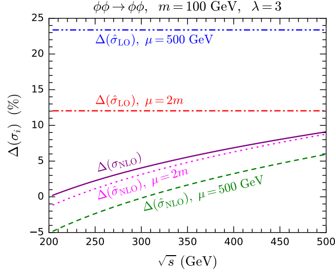
图 12.6: 截面相对偏差 \Delta(\sigma_{\text{NLO}}) 、 \Delta(\hat{\sigma}_{\text{LO}}) 和 \Delta(\hat{\sigma}_{\text{NLO}}) 随质心能 \sqrt{s} 的变化曲线。
