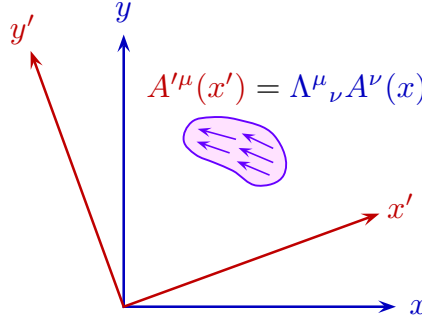
图 4.3: 在绕 z 轴空间旋转变换下, 矢量场 A^\mu(x) 的变换示意图。场的分布区域中的箭头示意性地代表矢量场的方向。
