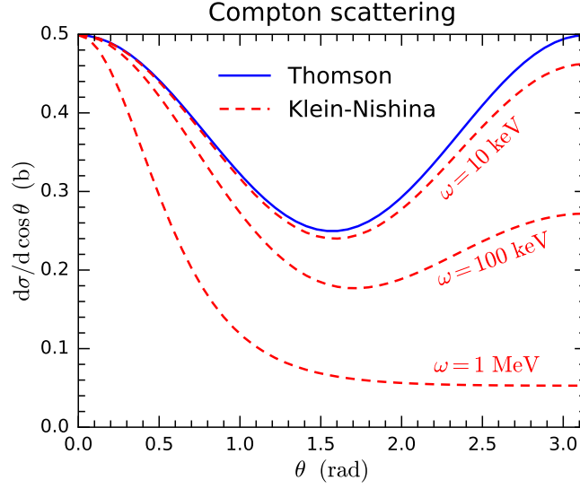
图 8.14: Thomson 公式和 Klein-Nishina 公式给出的微分散射截面随散射角 \theta 的变化。
