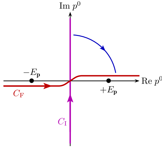
图 11.4: 将沿虚轴的积分路径 C_I 变形为路径 C_F 。
