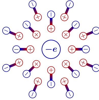
图 12.8: Q_{f'} = -1 时真空极化的经典图像。
