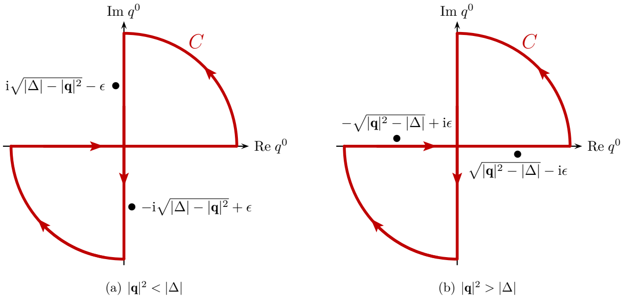
图 12.2: \Delta < 0 时, q^0 复平面上的极点位置和闭合曲线 C 。
