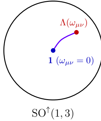
图 4.1: 固有保时向 Lorentz 群中的有限 Lorentz 变换 \Lambda(\omega_{\mu\nu}) 。
