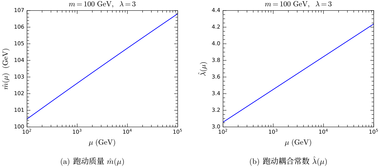
图 12.5: \hat{m}(\mu) 和 \hat{\lambda}(\mu) 随重整化能标 \mu 的跑动行为。
