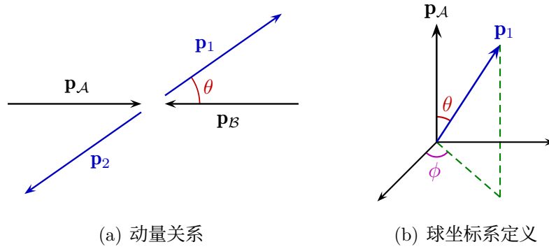
图 6.5: 质心系中 2 \rightarrow 2 散射过程的运动学示意图。
