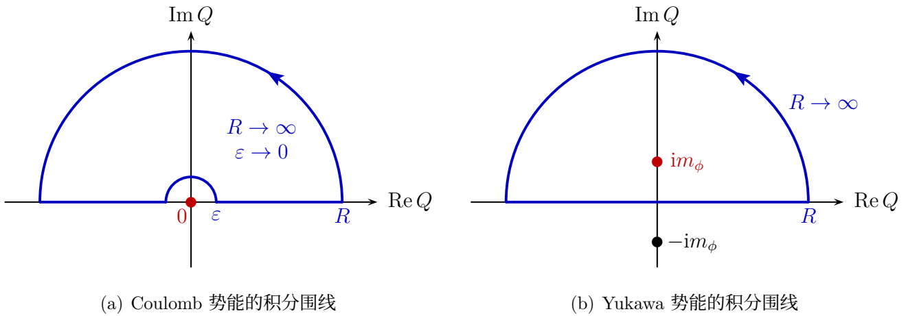
图 8.9: 计算 Coulomb 势能和 Yukawa 势能时使用的积分围线。
