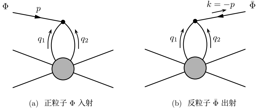
图 8.11: 交叉对称性示意图。
