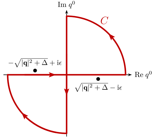
图 12.1: q^0 复平面上的闭合曲线 C 。这是示意性的, C 里面的圆弧实际上位于无穷远处。
