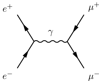
图 8.1: e^+ e^- \rightarrow \mu^+ \mu^- 领头阶 Feynman 图。
