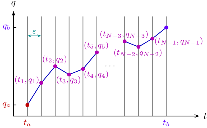
图 11.1: 连接 (t_a, q_a) 和 (t_b, q_b) 两点的一条路径。
