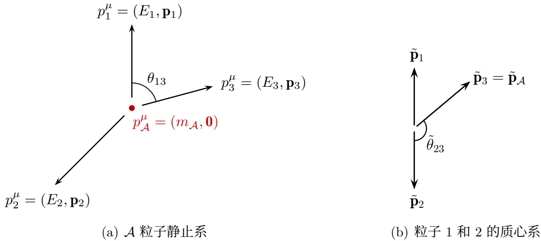
图 6.6: 三体衰变过程的动量示意图, 箭头指示三维动量的方向。
