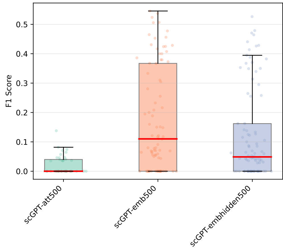
TF-level F1 Score Distribution
