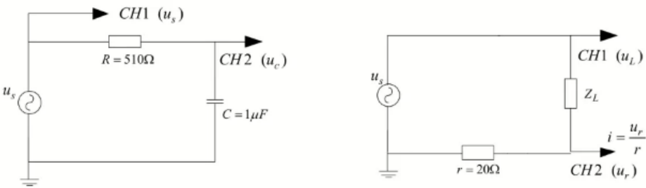
图 1: RC 电路相位差测量电路图
