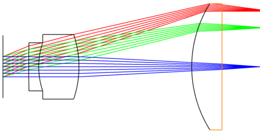
图 1: 凯尔纳目镜光路结构示意图 (Zemax 2D 布局图, 初始结构)
